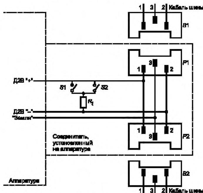
Рисунок Е.1 — Схема подключения аппаратуры к шине D2B
