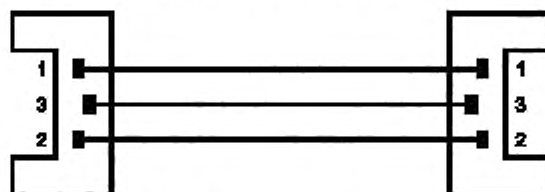
Рисунок Е.2 — Схема соединений кабеля шины
