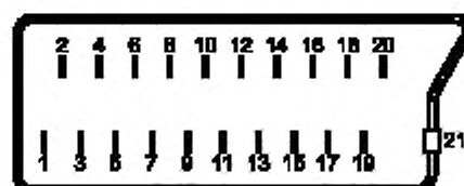
Рисунок В.1 — Расположение и нумерация контактов соединителя
