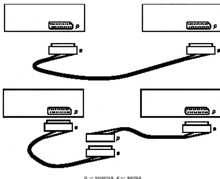
Рисунок Г.1 — Виды соединительных шнуров
