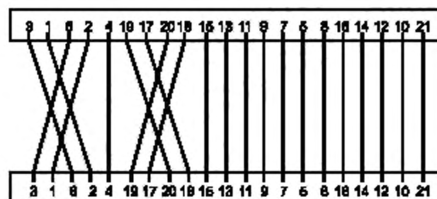
Рисунок В.3 — Кросс-соединения в шнурах аппаратуры с одинаковыми типами соединителей на концах шнура
