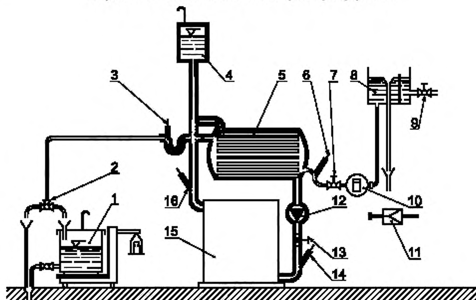
Рисунок И.1 — Испытательный стенд с прямой рециркуляцией
