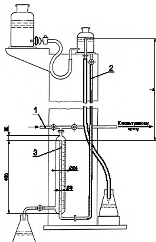
1 — сжатый воздух; 2 — градуированная шкала; 3 — измерительный сосуд
