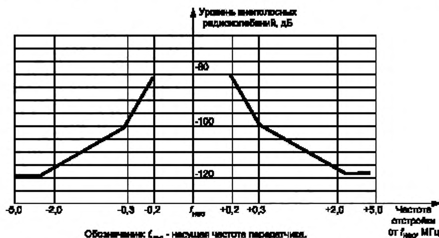
Рисунок 1 — Нормы внеполосных радиоколечаний
