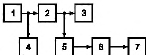
1 — генератор сигналов НЧ; 2 — передатчик; 3 — эквивалент антенны; 4 — милливольметр НЧ; 5 — элемент связи; 6 — девиометр; 7 — ИНИ или анализатор спектра НЧ
