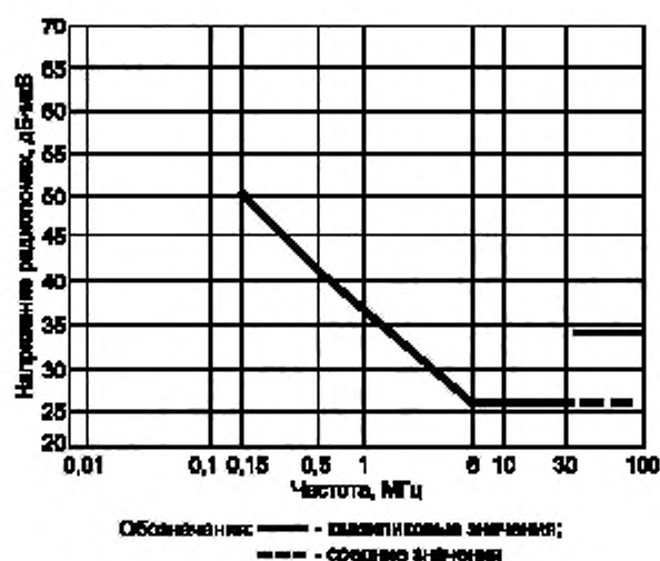
Рисунок 2 — Нормы напряжения радиопомех
