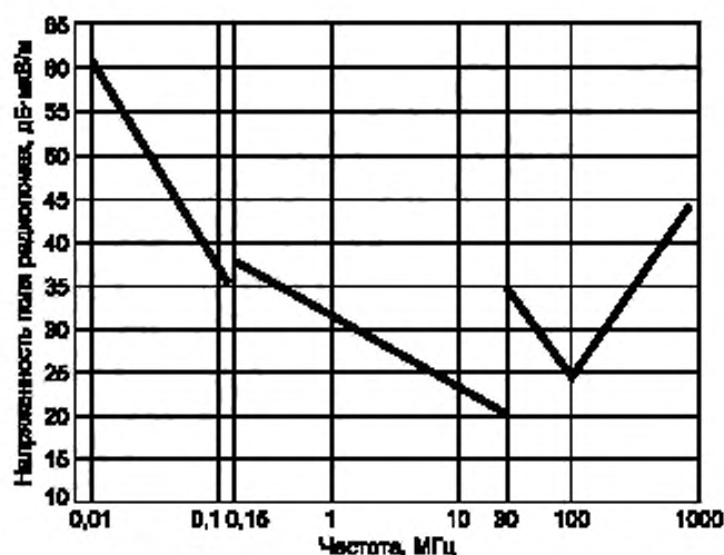
Рисунок 3 — Нормы напряженности поля радиопомех
