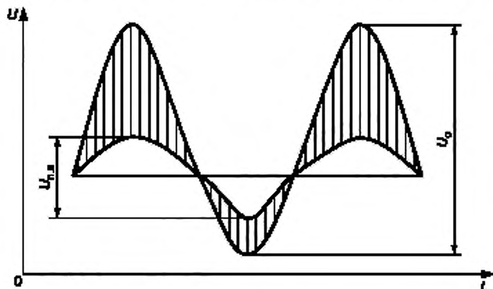
Рисунок 16а — Осциллограмма корреktированного КСС с переходной помехой на модулирующих частотах 1000 Гц и более
