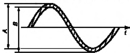
Рисунок 12 — Изображение сигнала в каналах А и В передатчика в режиме «Стереосигнал» (при синфазной модуляции)
