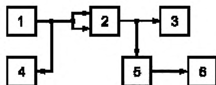
1 — генератор сигналов НЧ; 2 — передатчик; 3 — эквивалент антенны; 4 — милливольметр НЧ; 5 — элемент связи; 6 — девиометр
