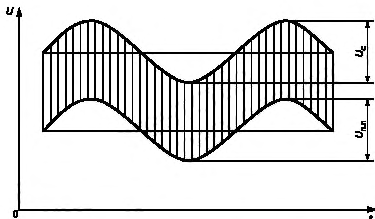
Рисунок 166 — Осциллограмма корреktированного КСС с переходной помехой на модулирующих частотах 100 Гц и менее
