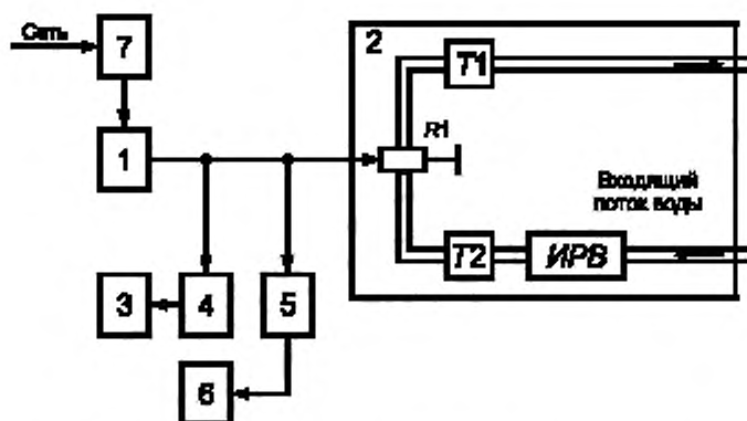
1 — передатчик; 2 — эквивалент антенны; R1 — водоохлаждаемый согласованный резистор; T1, T2 — термометры воды на выходе и входе системы охлаждения; ИРВ — измеритель расхода воды; 3 — частотомер; 4 — элемент связи; 5 — аттенюатор; 6 — вольтметр ВЧ; 7 — ваттметр
