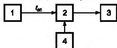
1 — возбудитель передатчика; 2 — частотный компаратор; 3 — частотомер; 4 — стандарт частоты; f_{\text{оп}} — опорная частота
