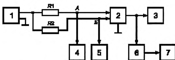
Рисунок 9 — Схема измерения коэффициента асимметрии симметричного НЧ входа
