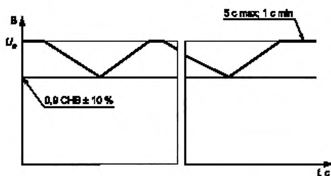
Рисунок 11 — Испытания на устойчивость функционирования при изменениях внешнего электропитания
