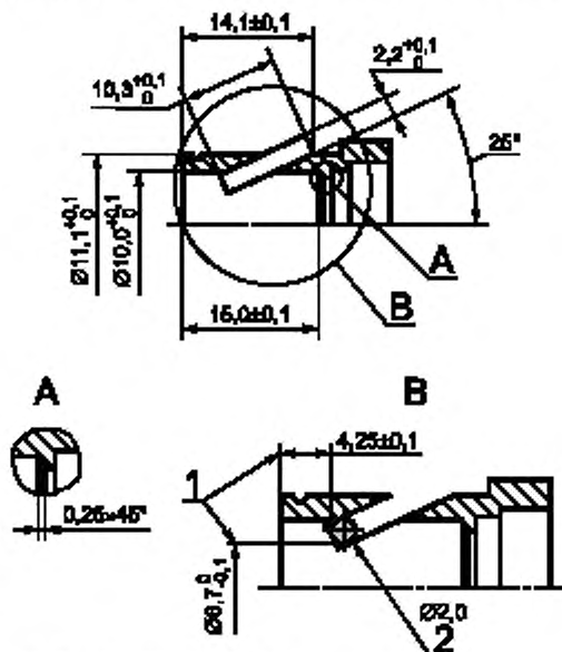
Рисунок 102 — АНЕСТЕЗИОЛОГИЧЕСКИЙ КОМПЛЕКС. ОБЩИЕ ВЫХОДНЫЕ ОТВЕРСТИЯ ГАЗА
