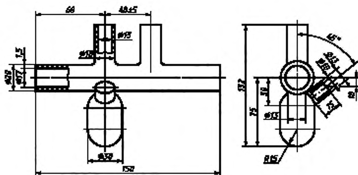
Рисунок Б.1 — Схема резервуара психрометра
