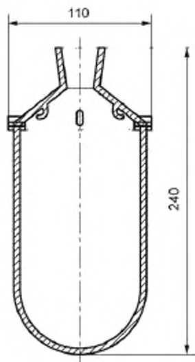
Рисунок 1 — Сосуд для проведения испытаний
