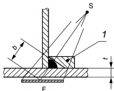
б) Схема контроля с кромочным компенсатором
