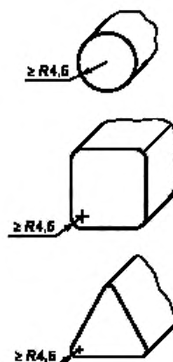
Рисунок 4 — Закругления деталей
