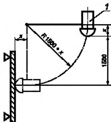
а) Горизонтальный удар по вертикальной поверхности
