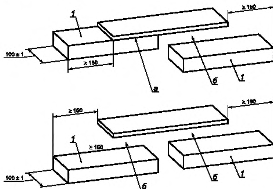
1 — верхнее покрытие мата безопасности с пеноматериалом; а — жесткий монтаж (сшивание, сварка и т.д.). б — разъемный монтаж (липучка, самоблокировка и т.д.)
