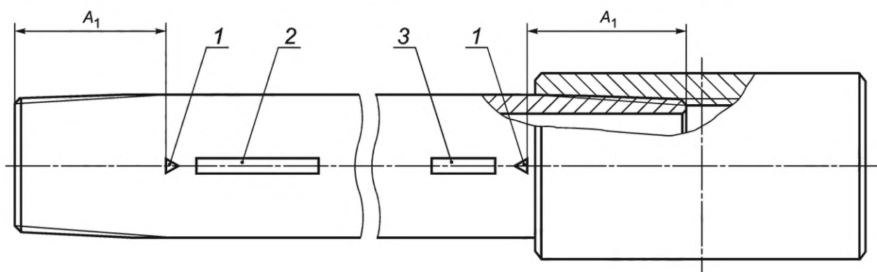
1 — треугольное клеймо; 2 — полоса размером 25 × 610 мм на nipple-конец трубы; 3 — полоса размером 25 × 102 мм на муфтовом конце трубы; A_1 — расстояние от торца трубы до основания треугольного клейма
