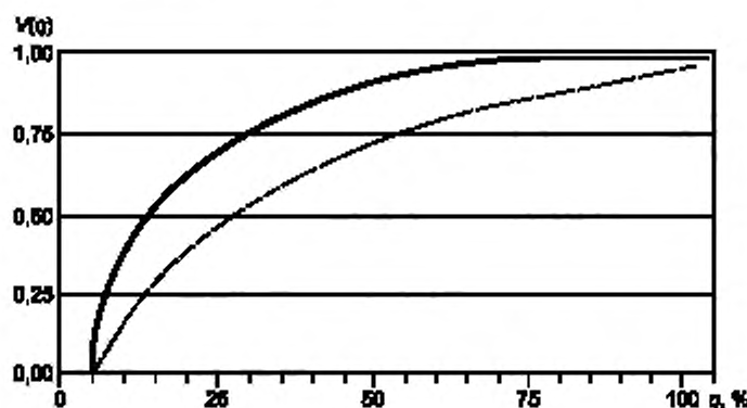
Рисунок Д.3 — Изменение выявляемости, определенной по формуле (Д.1) в зависимости от дефектности реальных объектов (зон) контроля в конкретной выборке
