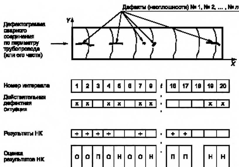
Рисунок Е.1 — Пример процедуры сравнения результатов НК с действительной дефектной ситуацией для расчета показателей достоверности результатов контроля
