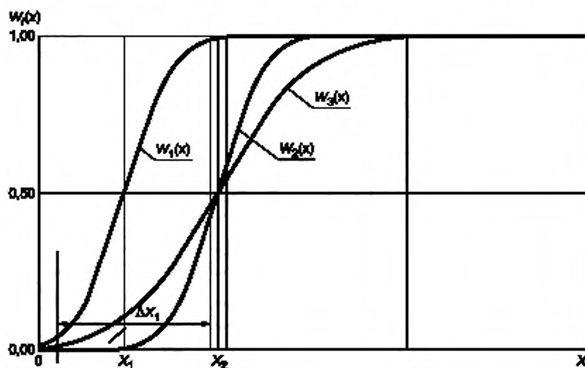
W_1(x) — кривая выявляемости для размера дефекта x_1 , \Delta x_1 — величина интервала выявляемых дефектов для размера x_1 , W_2(x) — кривая выявляемости для размера дефекта x_2 , W_3(x) — кривая выявляемости для размера дефекта x_2 по методике контроля, отличной от той, для которой построена кривая W_2(x) .
