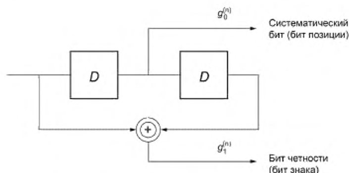
Рисунок 13 — Систематический сверточный кодировщик
