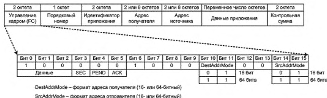
Рисунок 21 — Кодирование кадра данных
