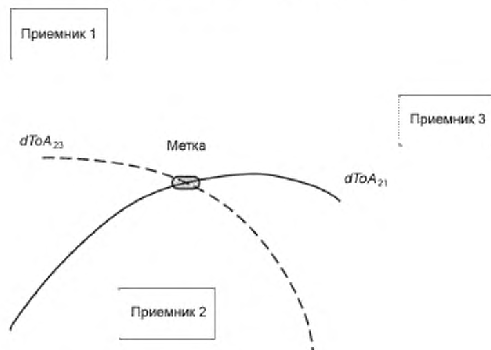
Рисунок A.4 — Определение местонахождения метки методом трилатерации
