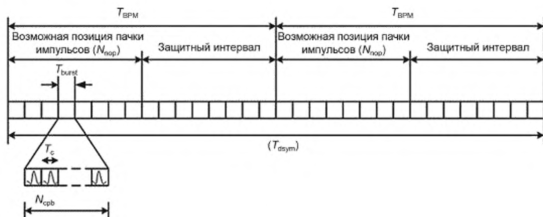
Рисунок 5 — Структура символа
