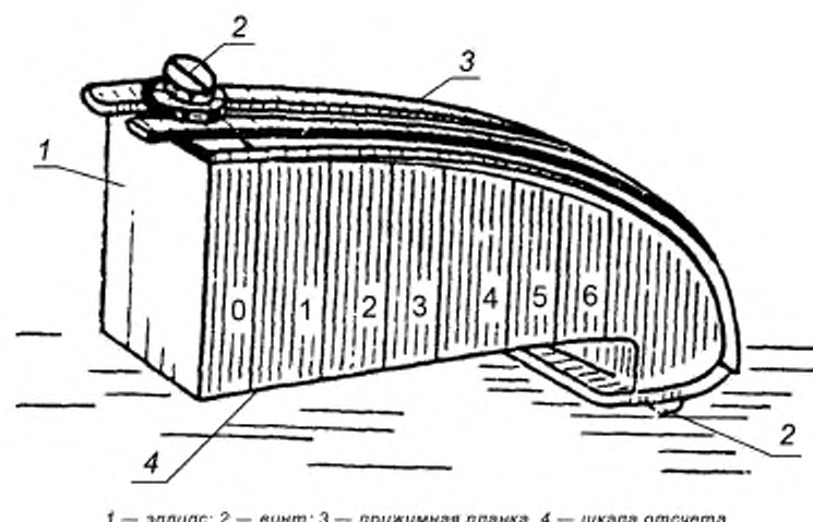
Рисунок 2 — Приспособление для создания напряженно-деформированного состояния
