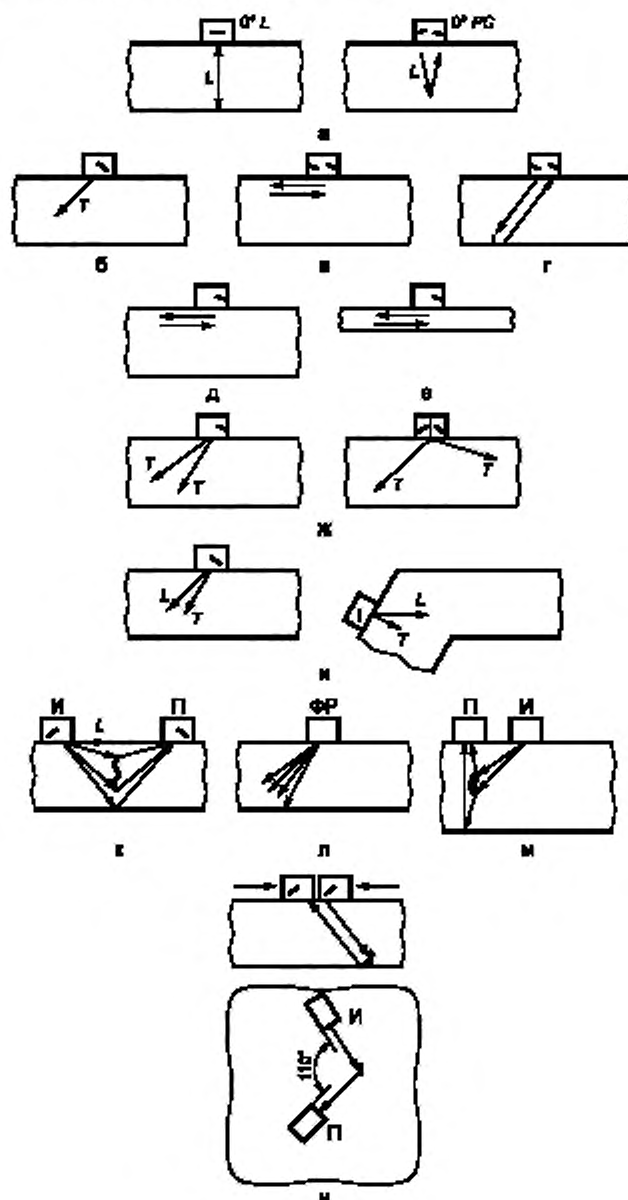
Рисунок 1 — Операции прозвучивания
