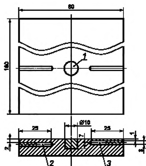
1 — вставка с несплошностью; 2, 3 — подповерхностные несплошности
