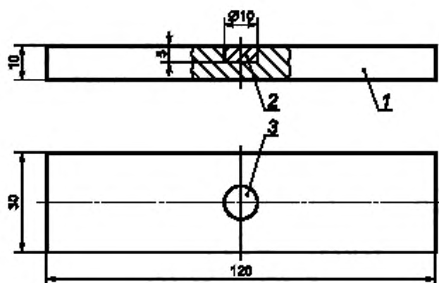
1 — брусок; 2 — вставка с несплошностью; 3 — подповерхностная несплошность
