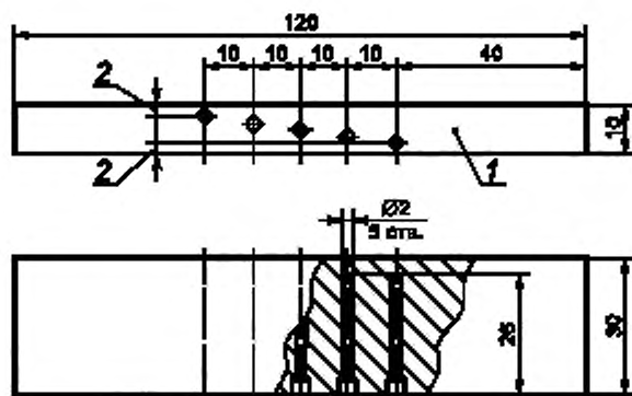
1 — брусок; 2 — цилиндрическое отверстие, закрытое винтом М 2,5
