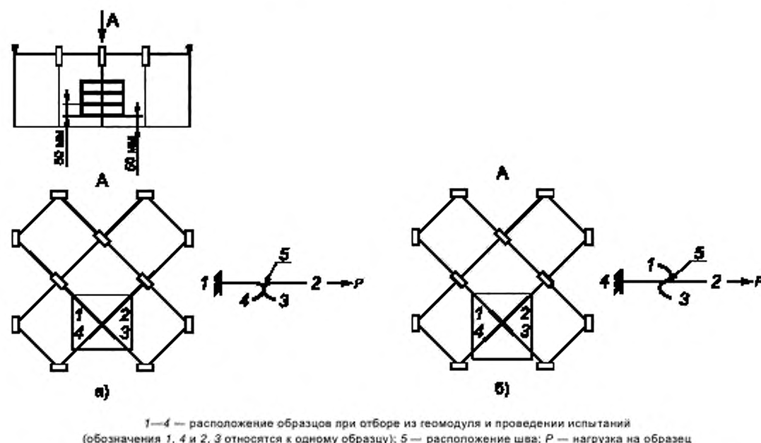
Рисунок А.1 — Отбор образцов для проведения испытаний по определению прочности шовных соединений геомодуля по схемам 1 (а) и 2 (б)
