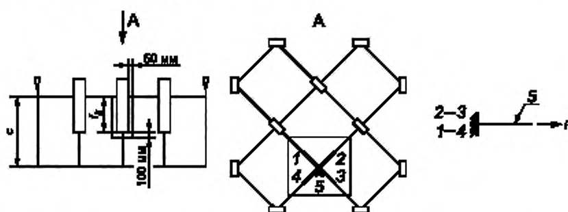
1—4 — расположение образцов при отборе из геомодуля и проведении испытаний (обозначения 1, 4 и 2, 3 относятся к одному образцу); 5 — расположение монтажной проушины; P — нагрузка на образец; c — высота ячейки; f_k — высота крепления монтажной проушины к ячейке геомодуля
