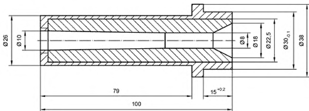
Рисунок 1 — Сопло для пескоструйной обработки
