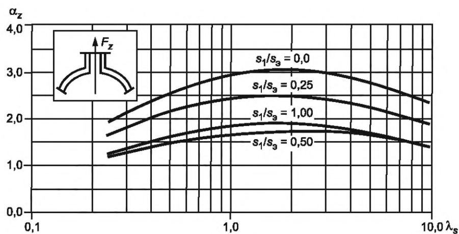
Рисунок Б.9 — Коэффициенты концентрации \alpha_z в месте пересечения штуцера со сферической оболочкой при осевом усилии на штуцер в зависимости от \lambda_s и отношения s_1/s_3
