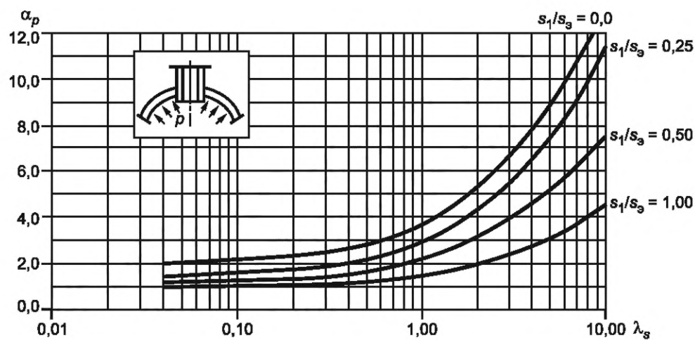
Рисунок Б.8 — Коэффициенты концентрации \alpha_p в месте пересечения проходящего штуцера со сферической оболочкой при внутреннем давлении в зависимости от \lambda_s и отношения s_1/s_2
