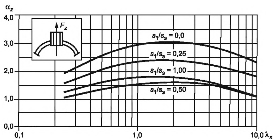
Рисунок Б.10 — Коэффициенты концентрации \alpha_z в месте пересечения проходящего штуцера со сферической оболочкой при осевом усилии на штуцер в зависимости от \lambda_s и отношения s_1/s_3
