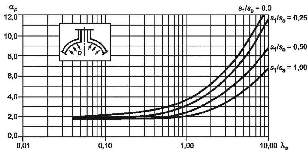
Рисунок Б.7 — Коэффициенты концентрации \alpha_p в месте пересечения штуцера со сферической оболочкой при внутреннем давлении в зависимости от \lambda_s и отношения s_1/s_2
