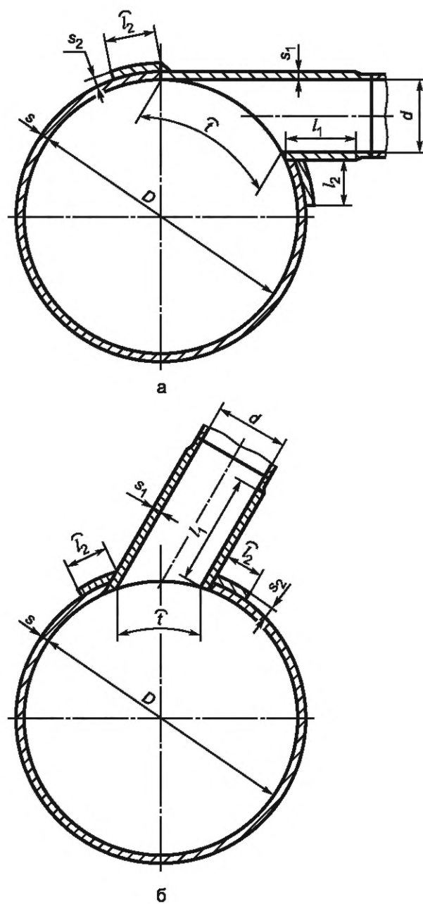
Рисунок А.12 — Наклонные штуцеры на обечайке в плоскости поперечного сечения
