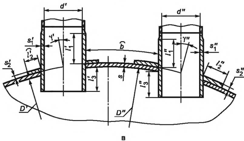
Рисунок А.8 — Укрепление взаимовлияющих отверстий
