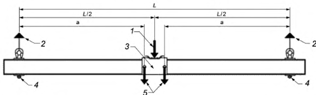
L — длина пролета; a — расстояние от оси сцепной арматуры до оси ближайшего болта центральной крепежной скобы; f — нагрузка при испытаниях; 2F; 2 — крепление траверсы за сцепную арматуру; 3 — центральная крепежная скоба; 4 — сцепная арматура; 5 — нагрузка на центральную крепежную скобу
