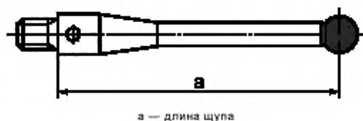
Рисунок 10 — Длина щупа
