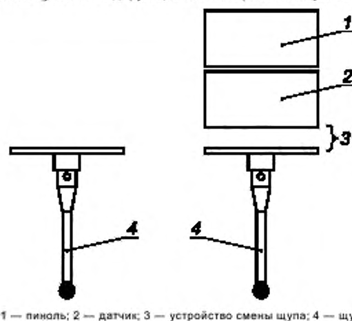
Рисунок 9 — Многощуповая зондирующая система (два одиночных щупа и устройство смены щупа)
