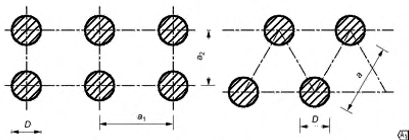
Рисунок 5 — Примеры группы свай
