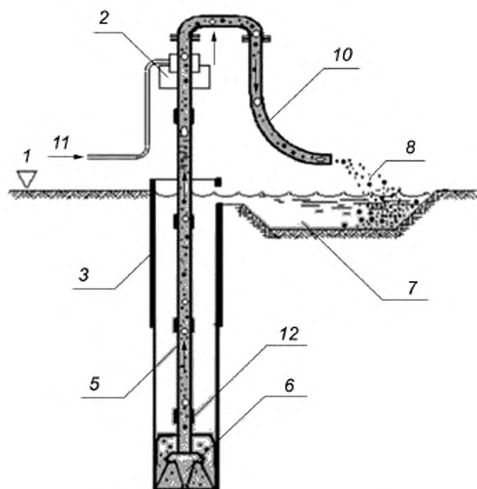
1 — уровень, с которого выполняется свая; 2 — привод, передающий момент на штангу; 3 — обсадная (направляющая) труба; 5 — буровая полая штанга для подъема потоком воздуха; 6 — буровая коронка; 7 — отстойник; 8 — буровой шлам, 10 — выпускной шланг; 11 — подвод воздуха в систему; 12 — подача воздуха в скважину
