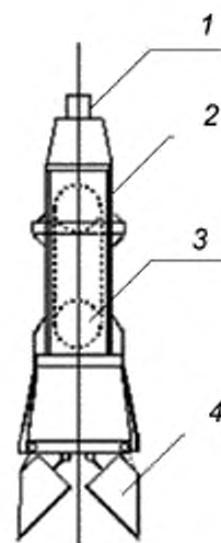
д) Буровой грейфер
