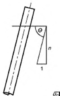
Рисунок 4 — Определение наклона свай
