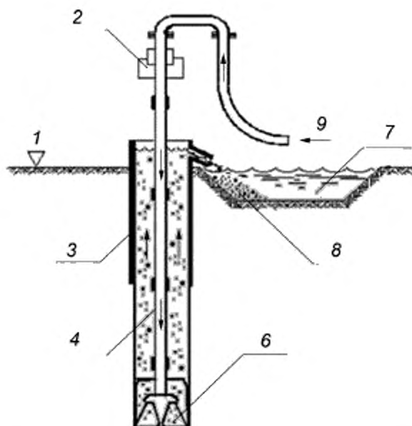
1 — уровень, с которого выполняется свая; 2 — привод, передающий момент на штангу; 3 — обсадная (направляющая) труба; 4 — буровая штанга; 6 — буровая коронка; 7 — отстойник; 8 — буровой шлам; 9 — шланг для соединения с насосом
