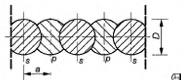
а) Баррета из буросекущих свай
