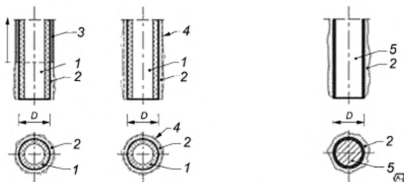
д) Свая из сборных железобетонных труб, заполняющихся бетоном, бентонитовым или цементным растворами
