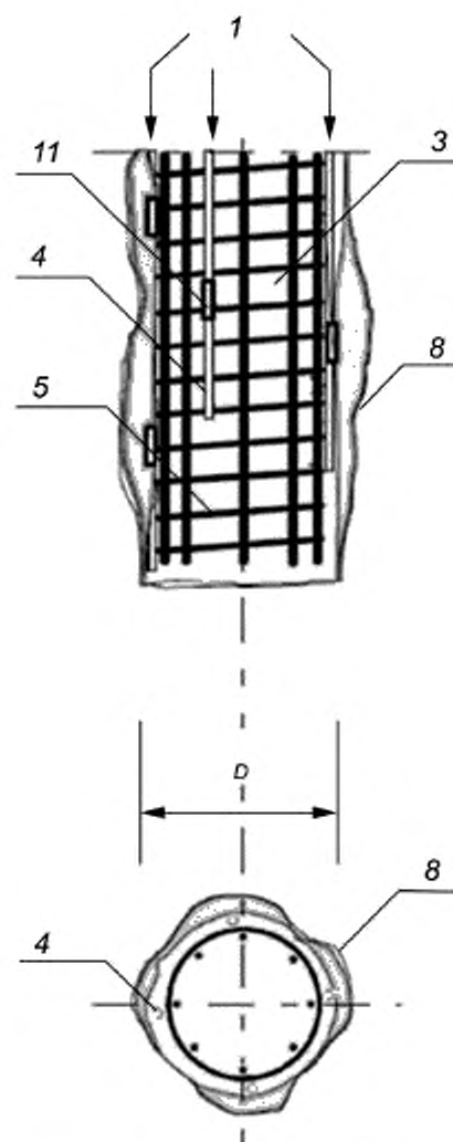
1 — опрессовка; 3 — скважина, заполненная бетоном; 4 — труба для опрессовки; 5 — арматурный каркас; 8 — нагнетаемый раствор; 11 — клапаны
