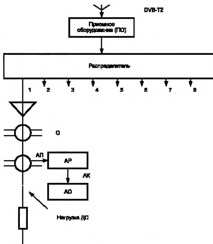
Рисунок А.1 — Система коллективного приема категории 1
