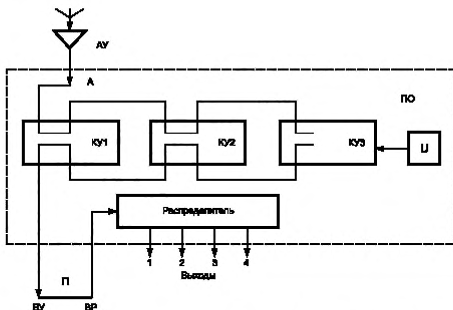
Рисунок А.3 — Приемное оборудование (ПО) системы коллективного приема
