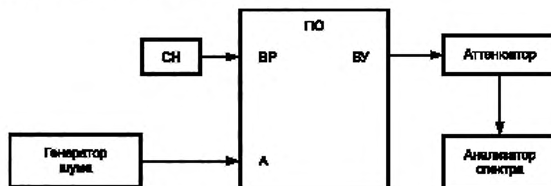
Рисунок 4 — Структурная схема для определения коэффициента шума приемного оборудования
