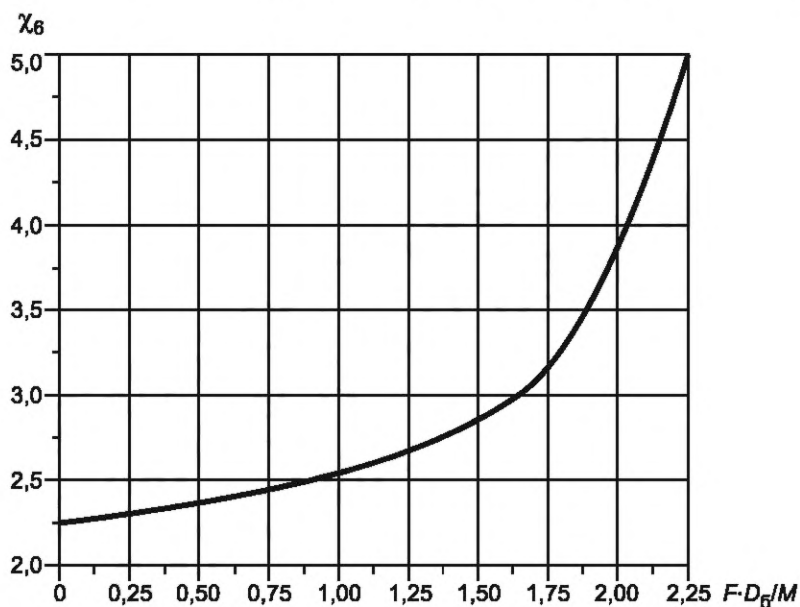
Рисунок 10 — Коэффициент \chi_6
