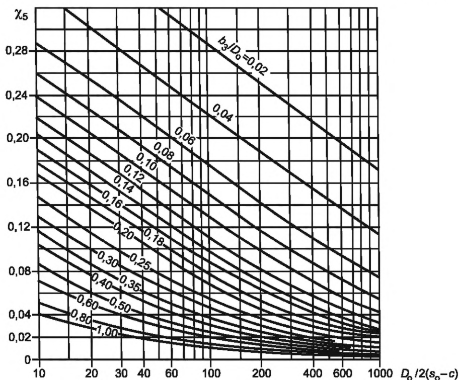
Рисунок 9 — Коэффициент \chi_5
