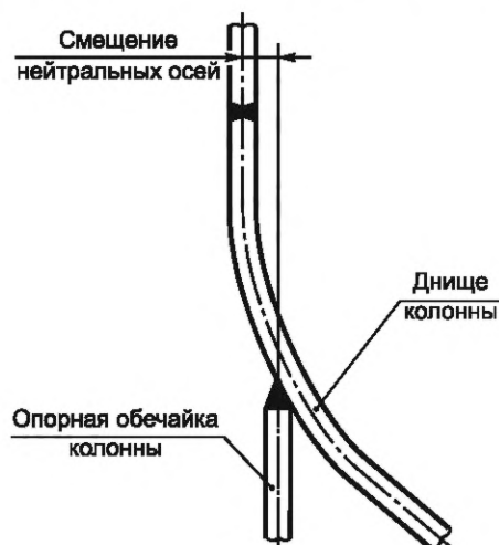
Рисунок 4 — Узел соединения опорной обечайки и днища аппарата
