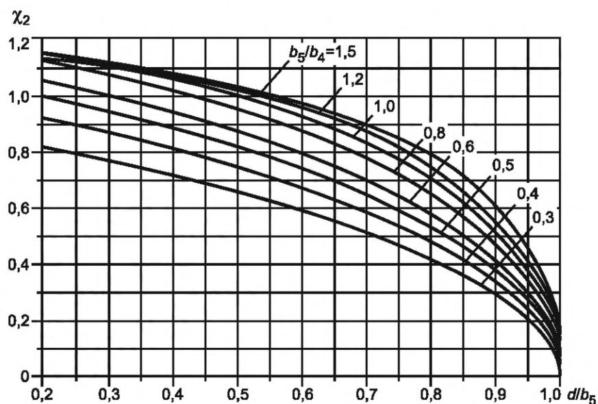
Рисунок 7 — Коэффициент \chi_2
