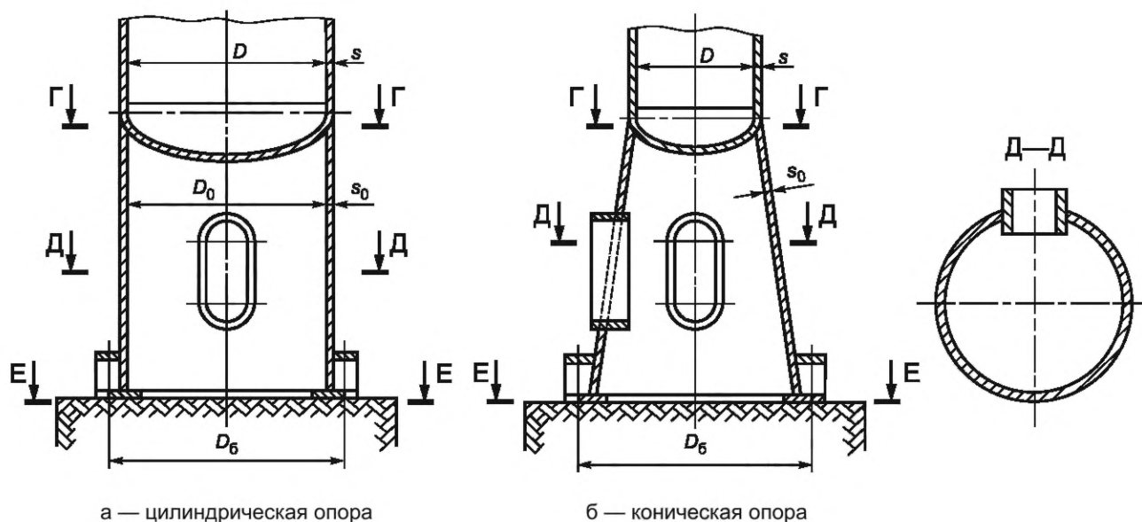
Рисунок 2 — Расчетные сечения опорной обечайки
