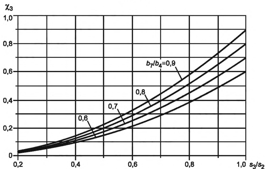
Рисунок 8 — Коэффициент \chi_3
