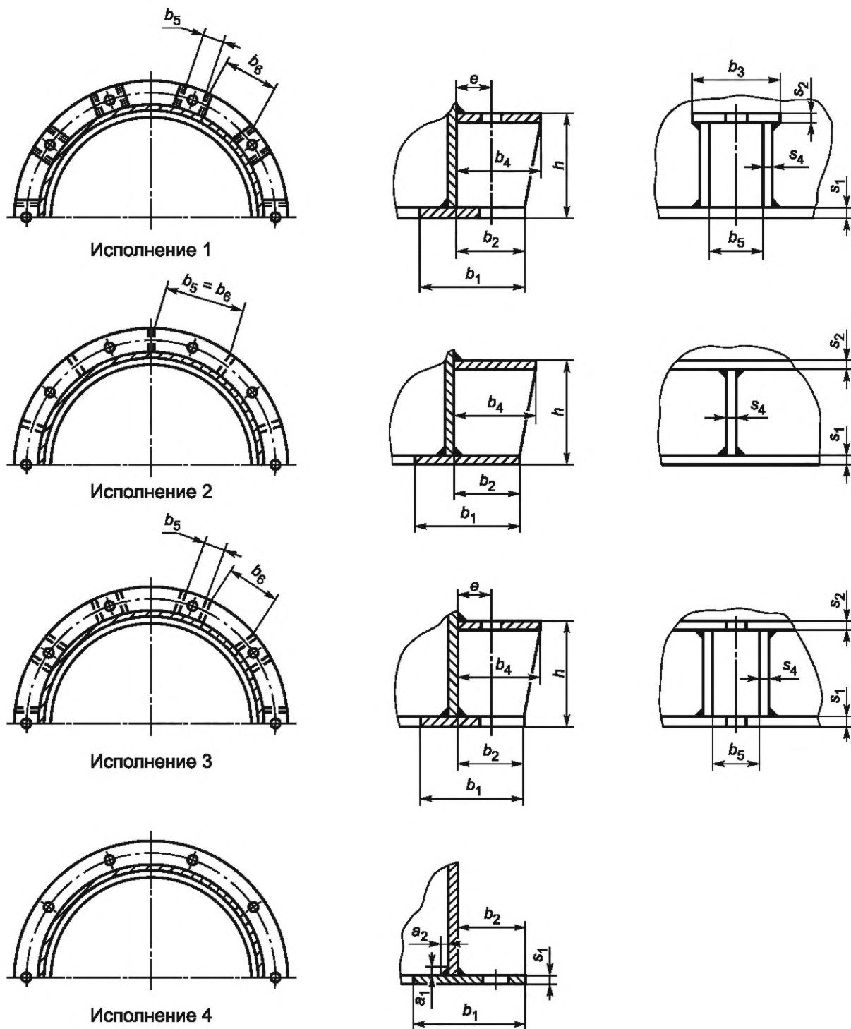
Рисунок 5 — Опорный узел
