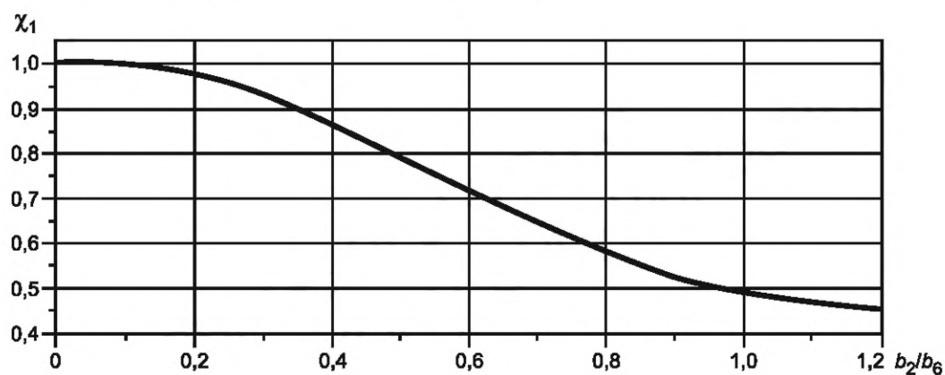
Рисунок 6 — Коэффициент \chi_1
