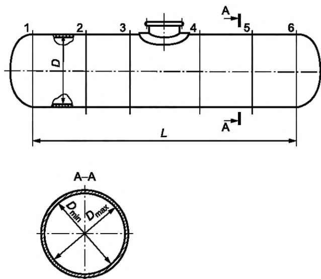
Эскиз № 1 к разделу 6 — «Карта измерений корпуса сосуда»
