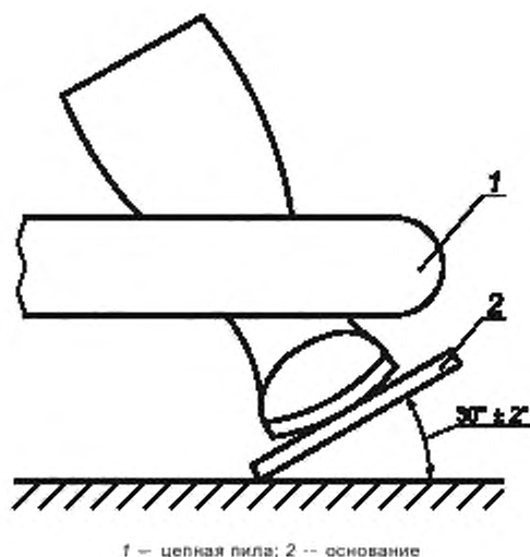
Рисунок 4 — Схема испытания в области союзки
