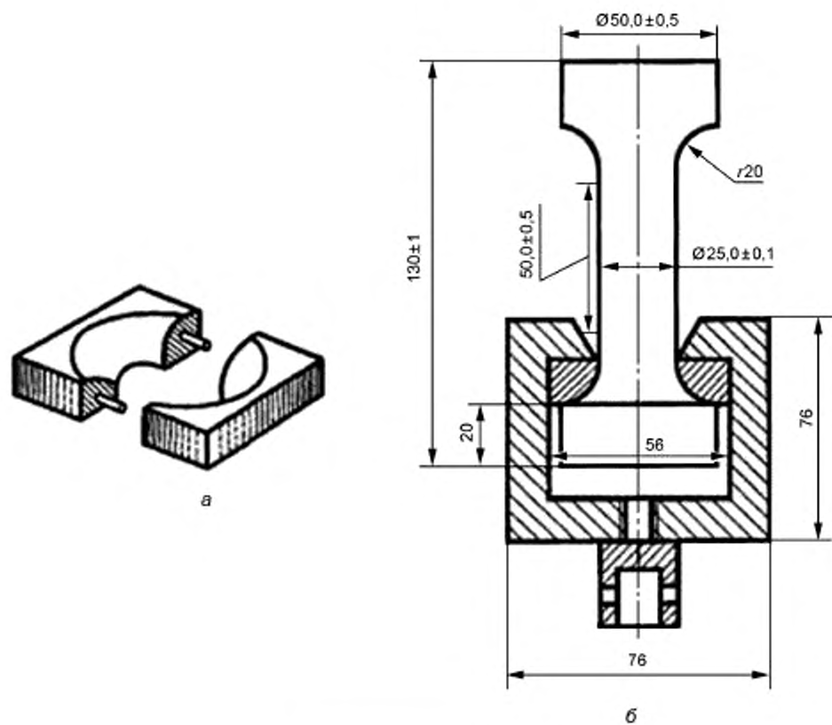
Рисунок 2 — Образец для испытания типа 2
