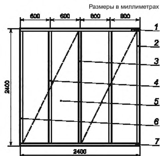
1 — верхнее ребро; 2 — крайнее ребро на стороне, противоположной стороне приложения нагрузки; 3 — среднее ребро; 4 — промежуточные ребра; 5 — деревянная обшивка из двух плит шириной 1200 мм, состыкованных на центральном ребре; 6 — крайнее ребро со стороны приложения нагрузки; 7 — нижнее (опорное) ребро
