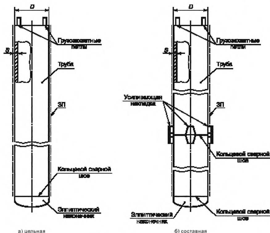
Рисунок 2 — Общий вид буропускной сваи
