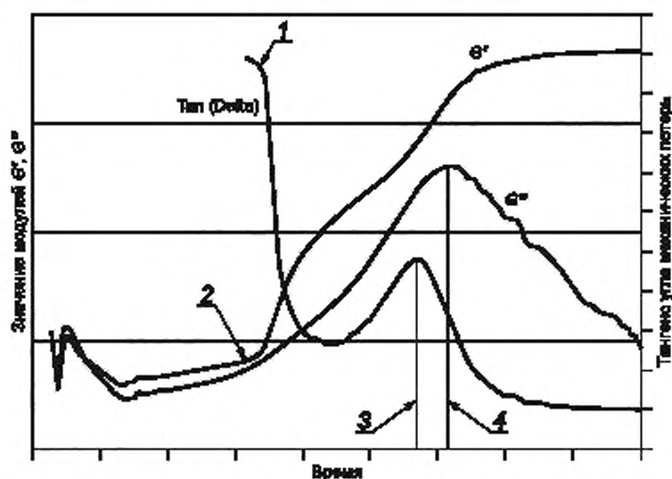
1 — время, когда значение тангенса угла механических потерь начинает быстро снижаться; 2 — время, когда значение модуля упругости G' резко возрастает; 3 — время достижения пика тангенса угла механических потерь, 4 — время достижения пика модуля потерь G''
