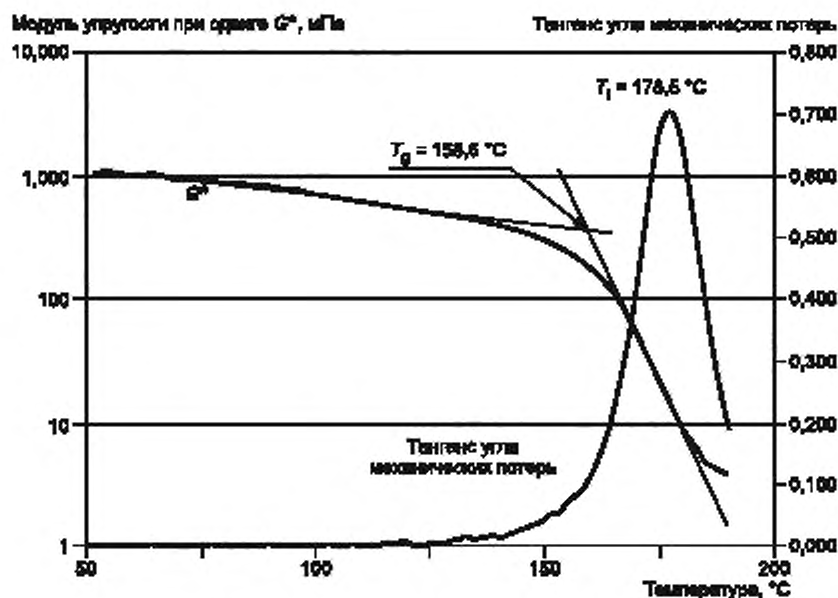
Рисунок 8 — Динамические методы определения температуры стеклования T_g после отверждения или T_c линейным изменением температуры
