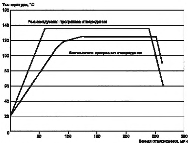
Рисунок 2 — Стандартная температурная программа отверждения компонентов и фактическая температура при отверждении
