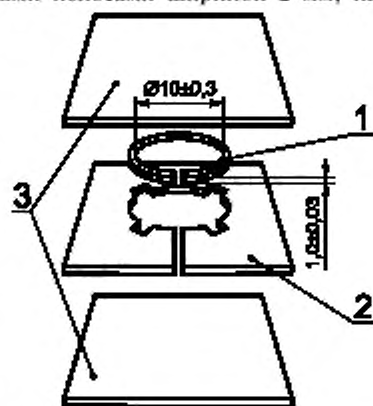
1 — расщепленное кольцо; 2 — удерживающая пластина; 3 — покровные пластины
