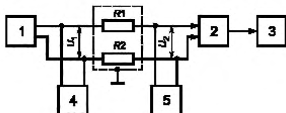
1 — генератор сигналов НЧ; 2 — передатчик; 3 — эквивалент антенны; 4, 5 — вольтметры НЧ; R1 , R2 — резисторы сопротивлением (300 \pm 1,5) Ом
