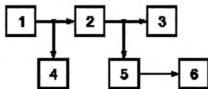
1 — генератор сигналов НЧ; 2 — передатчик; 3 — эквивалент антенны; 4 — милливольметр НЧ; 5 — элемент связи; 6 — модулометр
