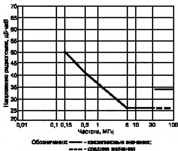
Рисунок 1 — Нормы напряженности радиопомех
