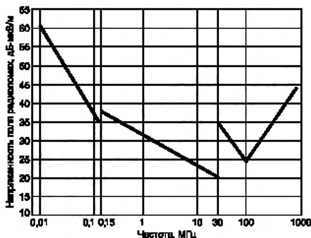
Рисунок 2 — Нормы напряженности поля радиопомех
