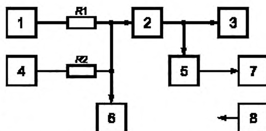
1 — генератор сигналов НЧ; 2 — передатчик; 3 — эквивалент антенны; 4 — генератор сигналов НЧ; 5 — элемент связи; 6 — милливольтметр НЧ; 7 — модулятор; 8 — анализатор спектра ВЧ; R1, R2 — резисторы сопротивлением (6,8 \pm 0,34) \text{ кОм}
