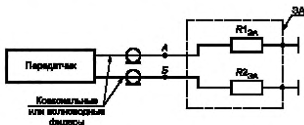
Рисунок Г.1 — Схема измерения мощности передатчика с симметричным ВЧ выходом
