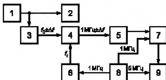
Рисунок 6 — Схема измерения отклонения рабочей частоты от номинального значения для передатчиков синхронного вещания
