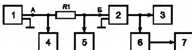
1 — генератор сигналов НЧ; 2 — передатчик; 3 — эквивалент антенны; 4, 5 — милливольтметры НЧ; 6 — элемент связи; 7 — модулятор; R1 — резистор сопротивлением (600 \pm 3) Ом
