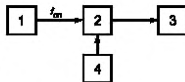
1 — возбудитель передатчика; 2 — частотный компаратор; 3 — частотомер; 4 — стандарт частоты; f_{оп} — опорная частота
