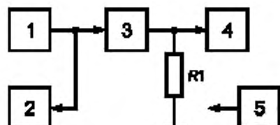
1 — генератор сигналов НЧ; 2 — милливольметр НЧ; 3 — возбудитель передатчика; 4 — милливольметр ВЧ; 5 — анализатор спектра ВЧ; R1 — резистор сопротивлением (75±4) Ом
