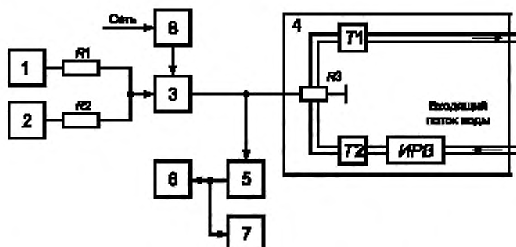
1, 2 — генераторы сигналов НЧ; 3 — передатчик; 4 — эквивалент антенны; R3 — водоохлаждаемый согласованный резистор; T1, T2 — термометры воды на выходе и входе системы охлаждения; ИРВ — измеритель расхода воды; 5 — элемент связи; 6 — анализатор спектра ВЧ; 7 — осциллограф; 8 — ваттметр (измерительный комплект для измерения потребляемой мощности); R1, R2 — резисторы сопротивлением (6,8±0,34) кОм
