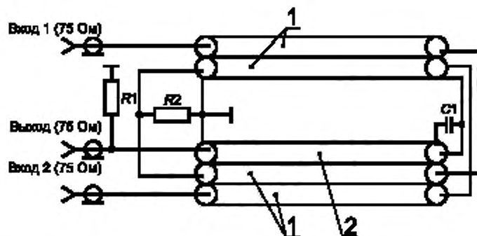
Рисунок Г.2 — Электрическая схема сумматора противофазных сигналов
