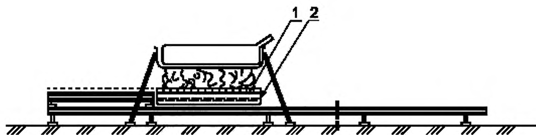
Рисунок 3 — Фаза С. Воздействие пламени на некотором расстоянии
