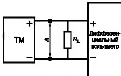
Рисунок 4 — Схема измерения выходного шума ТМ
