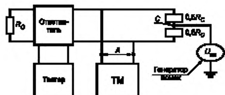
Рисунок 7 — Схема тестирования входного сигнала при синфазных помехах и непосредственном подключении ТМ
