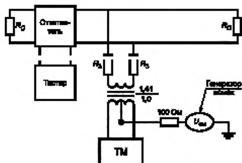
Рисунок 6 — Схема тестирования входного сигнала при синфазных помехах и трансформаторном подключении ТМ
