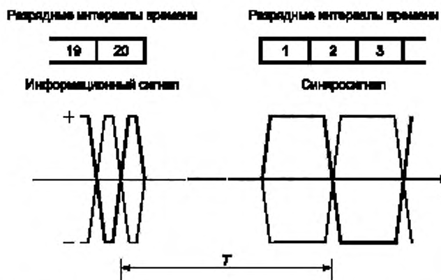
Рисунок 8 — Измерение времени паузы при передаче информации
