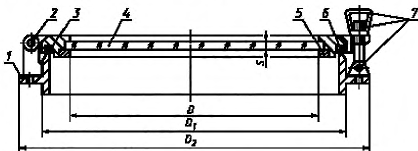
1 — корпус; 2 — петля; 3 — рама; 4 — стекло; 5 — резьбовое кольцо для крепления стекла; 6 — уплотнительная прокладка; 7 — задрайка (откидной болт, гайка-барашек, ось)
