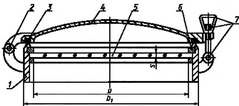
1 — корпус; 2 — петля; 3 — уплотнительная прокладка; 4 — штормовая крышка; 5 — стекло; 6 — резьбовое кольцо для крепления стекла; 7 — задрейка (откидной болт, гайка-барашек, ось)
