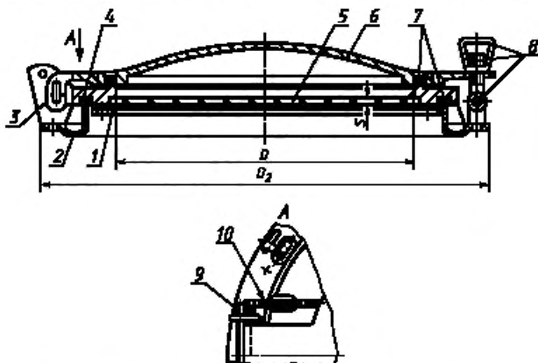
1 — кольцо на винтах для крепления стекла; 2 — корпус; 3 — петля; 4 — рама; 5 — стекло; 6 — штормовая крышка; 7 — уплотнительная прокладка; 8 — задрайка (откидной болт, гайка-барашек, ось); 9 — закладной штырь; 10 — цепочка
