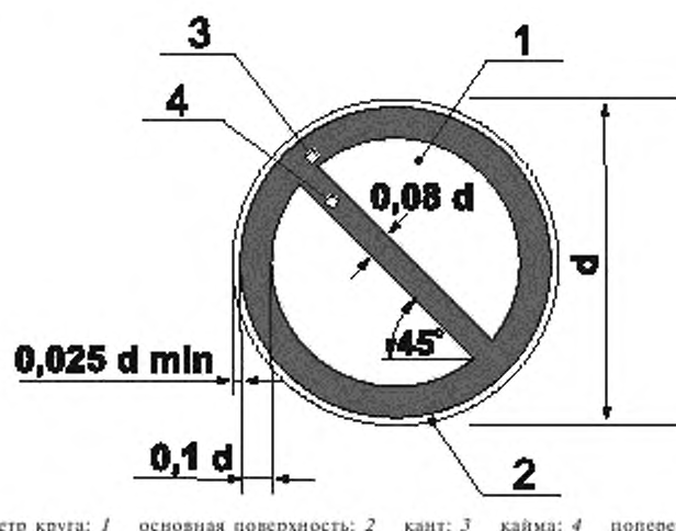
Рисунок 1 — Основа цветографического изображения и соотношение размеров запрещающих знаков безопасности
