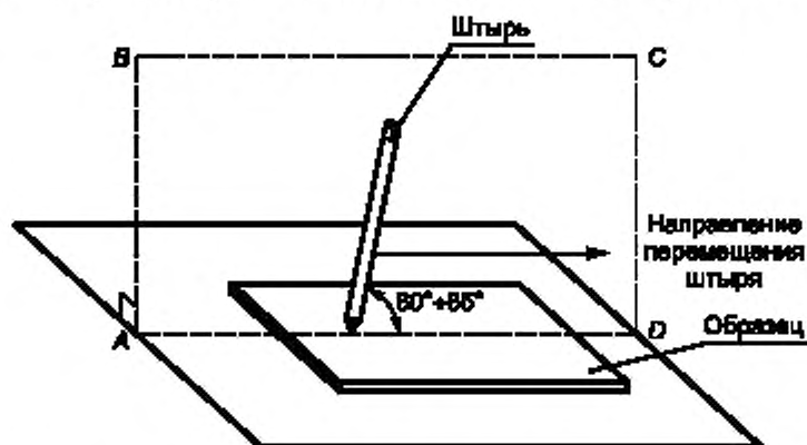
Рисунок 101 — Испытание на прочность покрытия ограждения царапанием
