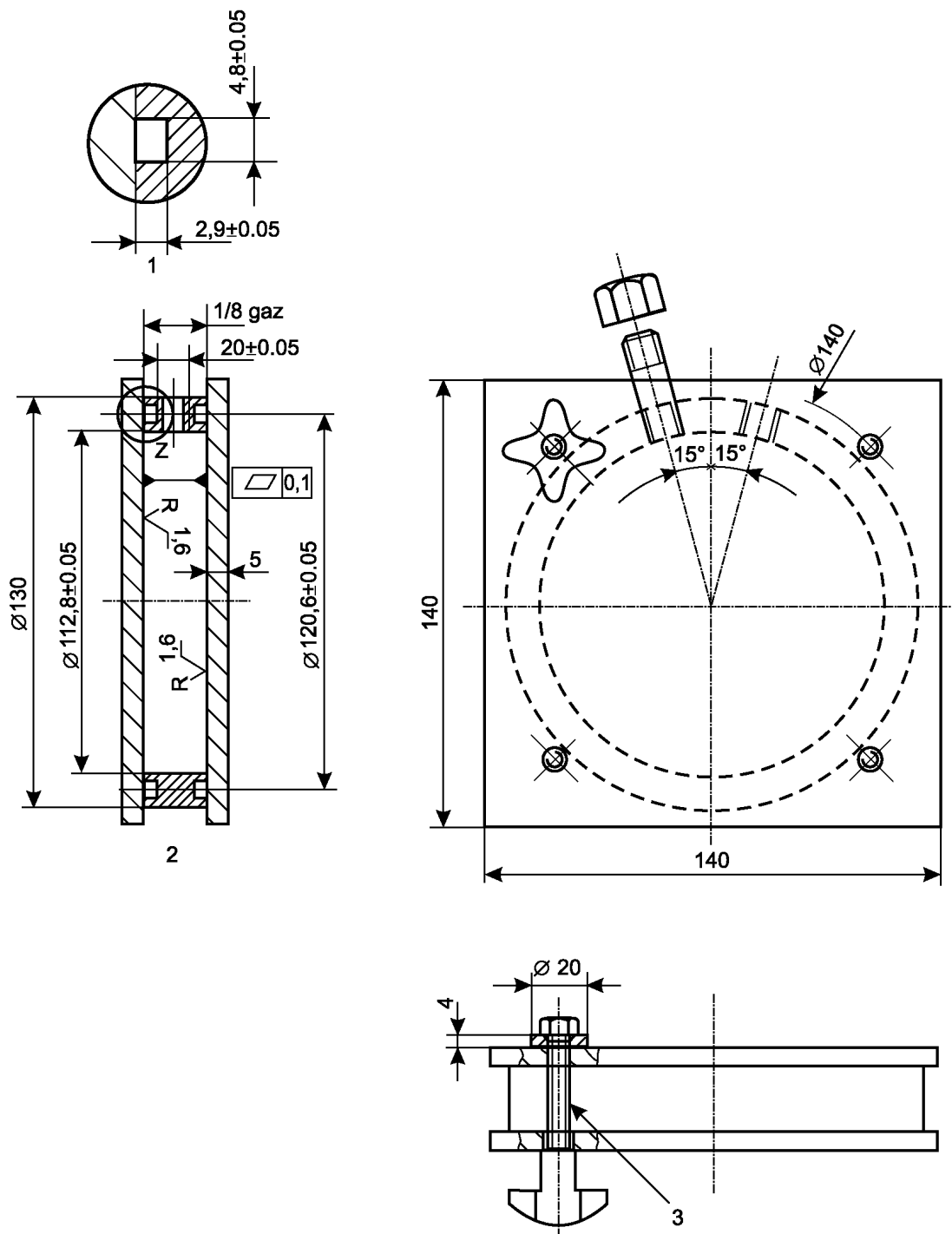
1 – деталь Z; 2 – уплотнительное кольцо \varnothing 117,07 / 124,13 / 3,53 ; 3 – винт НМФ-50
