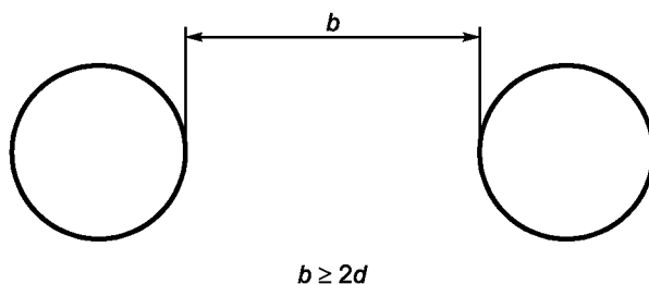
Рисунок 8 — Расположение двух отверстий
