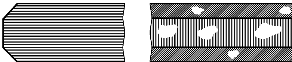
Рисунок 6, b — Грубо шлифованная кромка (есть необработанные участки)
