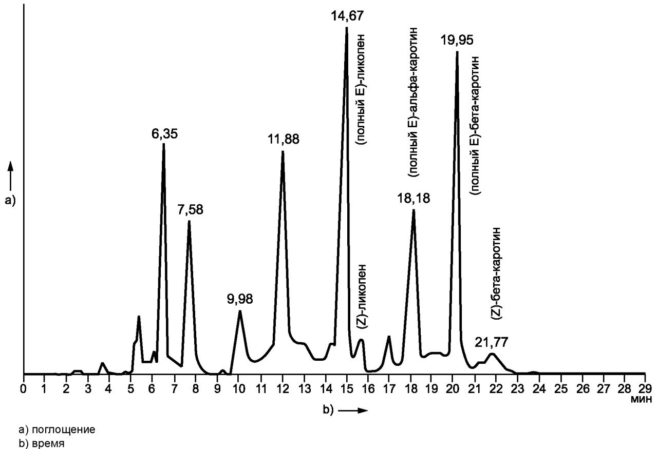
Рисунок А.1 — Пример хроматографического разделения \alpha и \beta -каротинов и ликопина в пробе овощной смеси
