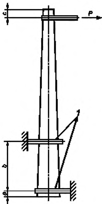
a — расстояние от торца секции до первого стропы, b — расстояние между удерживающими стропами; c — расстояние от торца секции до крепления тянущего троса (стропы); P — изгибающая сила, 1 — строп
