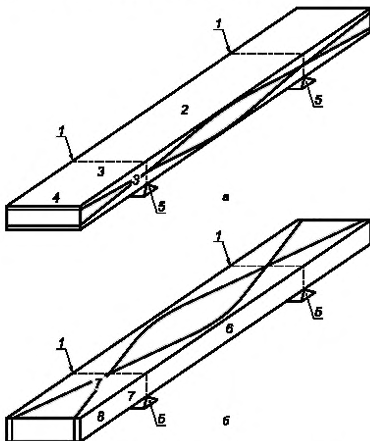
а — изгиб вне плоскости; б — изгиб в плоскости; 1 — узловая линия изгиба; 2 — точка импульса изгибающей вибрации вне плоскости; 3, 7 — точка установки контактного датчика; 4, 8 — точка установки бесконтактного датчика; 5 — опоры; 6 — точка импульса изгибающей вибрации в плоскости
