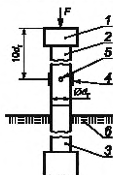
1 — наковальня; 2 — специально оборудованный участок штанг (инструментальная штанга); 3 — забивная штанга; 4 — тензорезистор (измерительный преобразователь); 5 — акселерометр; 6 — грунт; F — усилие; d_s — диаметр штанги
