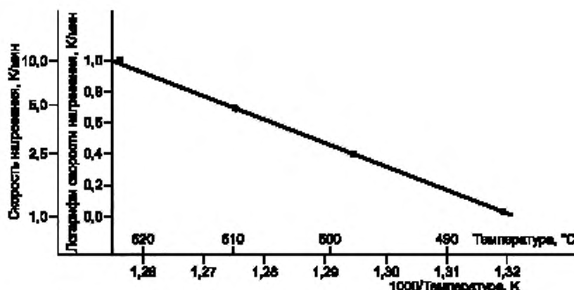
Рисунок 2 — График в координатах Аррениуса для скорости нагревания и температуры для данных постоянной степени превращения
