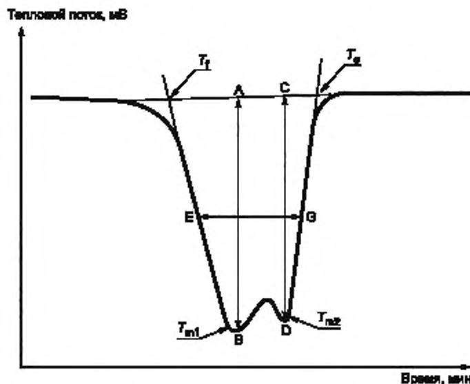
Рисунок 1 — ДСК-кривая нагрева
