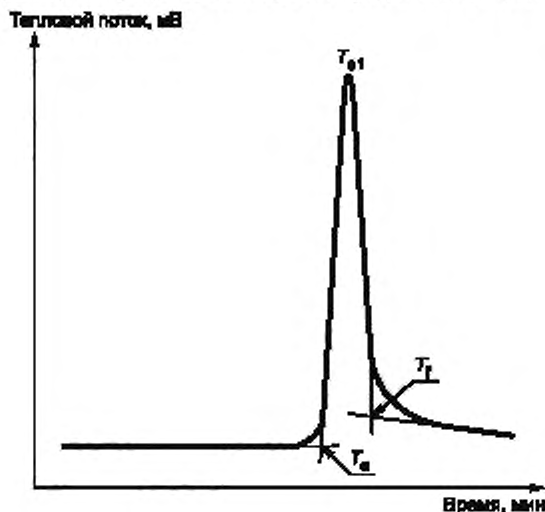
Рисунок 2 — ДСК-кривая охлаждения
