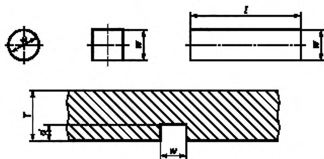
Рисунок 1 — Типы настроечных отражателей
