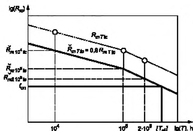
Рисунок А.1 — Диаграмма для определения [T_{ad}]
