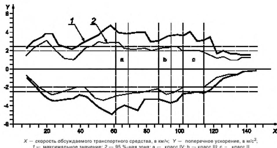
Рисунок 5 — Поперечное ускорение для среднего водителя
