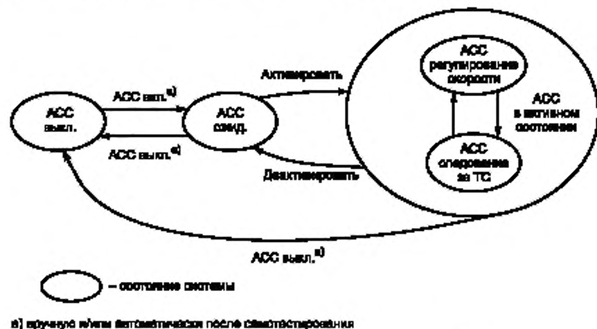
Рисунок 2 — Состояния и переходы системы ACC
