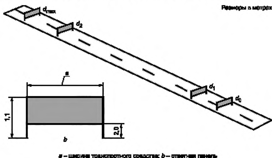
Рисунок 7 — Зона распознавания в продольном направлении
