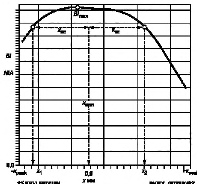
Рисунок 7 — Определение точки симметрии x_{\text{sym}} характеристики нелинейного коэффициента силы Bl(x)
