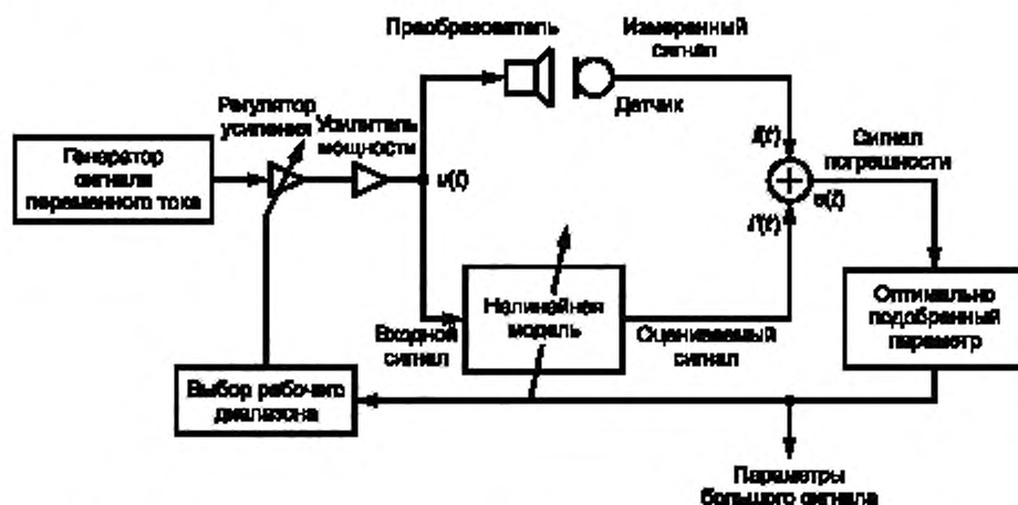
Рисунок 4 — Установка для динамического измерения параметров больших сигналов
