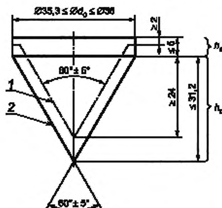
Рисунок 5 — Требования к допускам при применении наконечника
