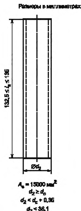
Рисунок 6 — Требования к допускам для муфты трения
