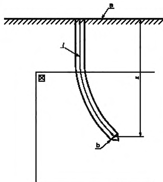
z — глубина зондирования, м; l — длина зондирования, м; a — неподвижная горизонтальная плоскость; b — основание конической части конуса
