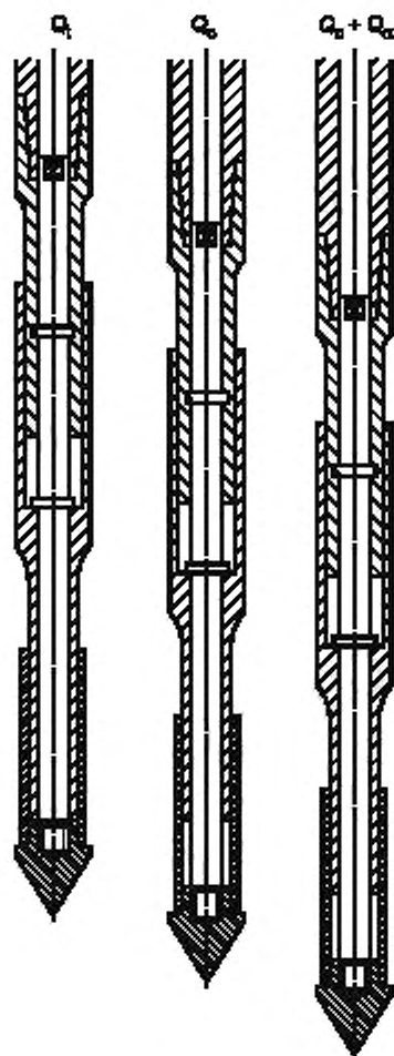
Рисунок 3 — Наконечник M2 (конус с кожухом, муфта трения)
